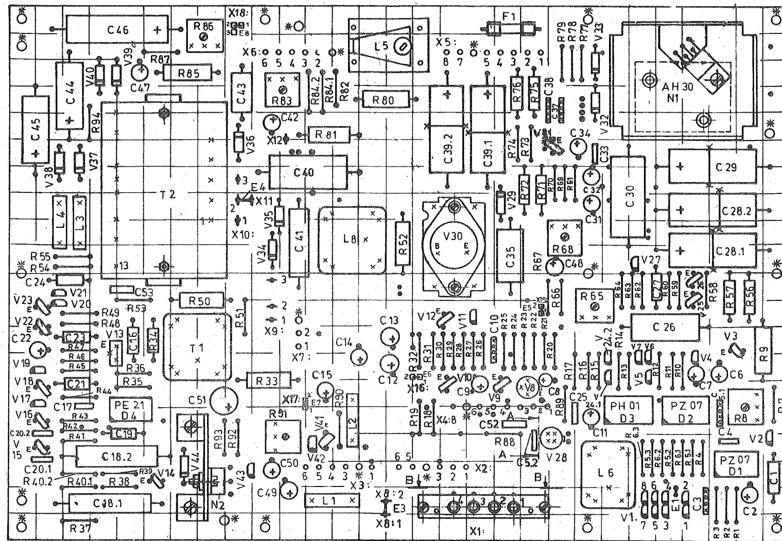
Leiterplatte, bstü Typ 013-1040 Belegungsplan
