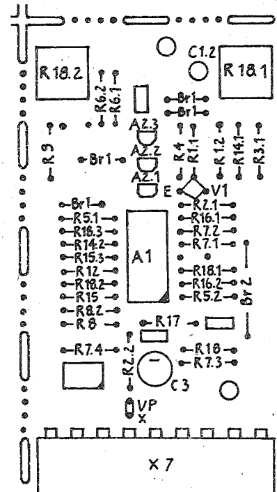
Leiterplatte bstü MSS TYP 062 - 9295 1.62.519295.5/09 G
