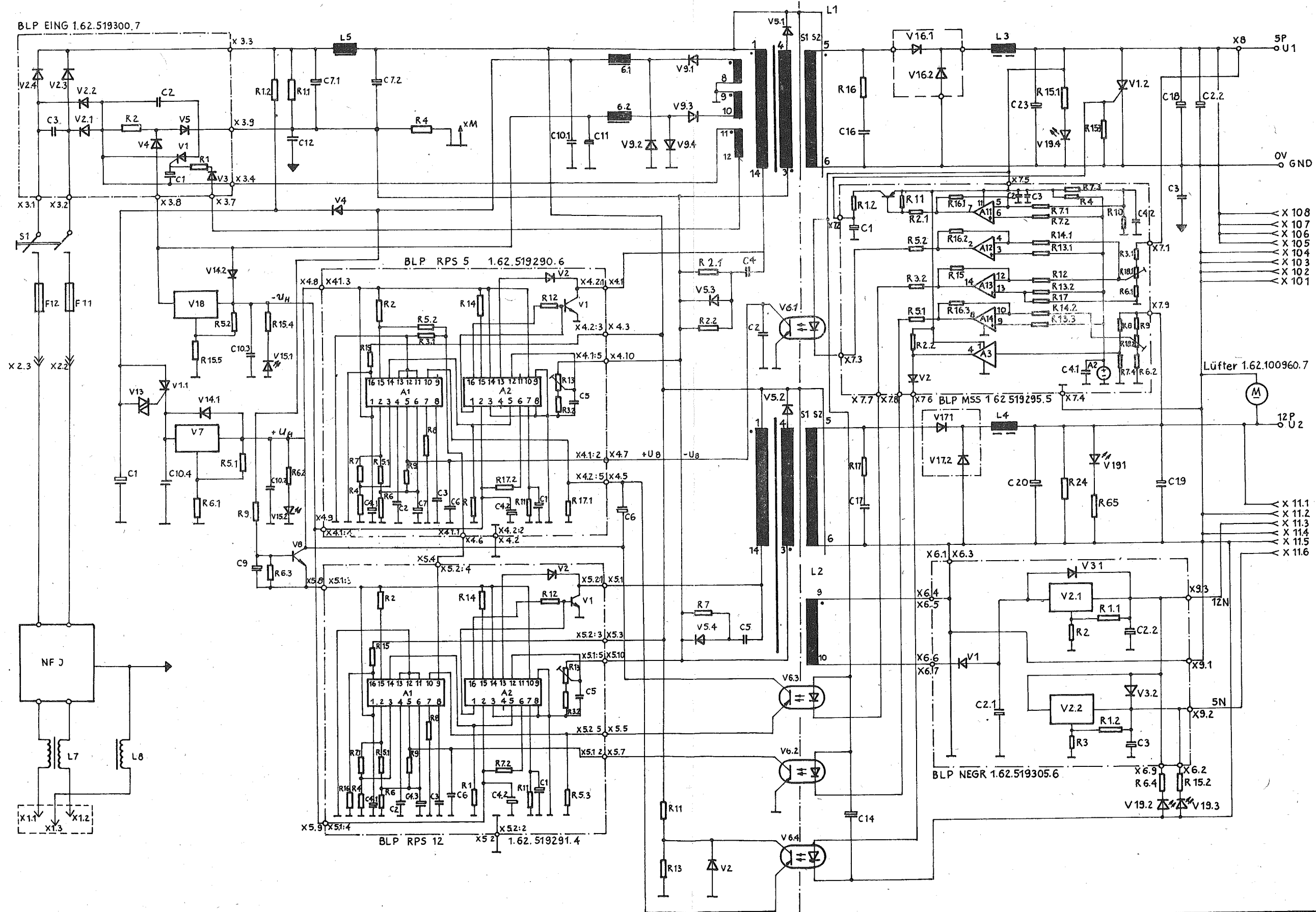
Stromversorgung Grundeinheit Gesamtstromlaufplan haus
