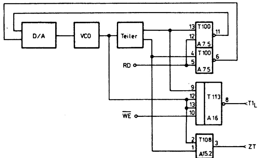
Abb. 9 Taktbildung Lesen
