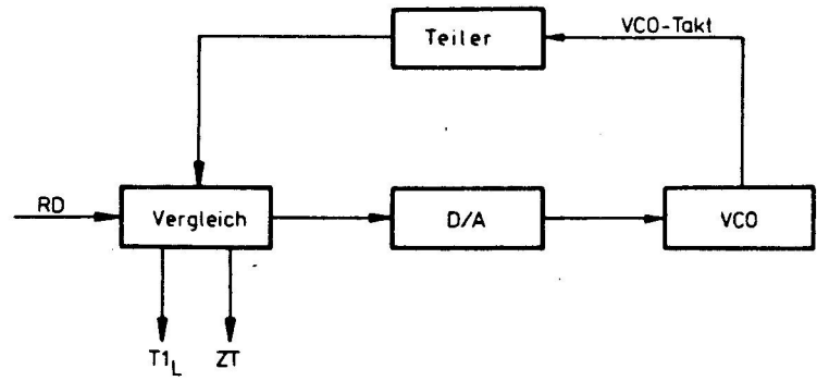
Abb. 8 Blockschaltbild PLL-Schaltung
