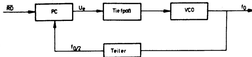
Abb. 1 Blockschaltbild
