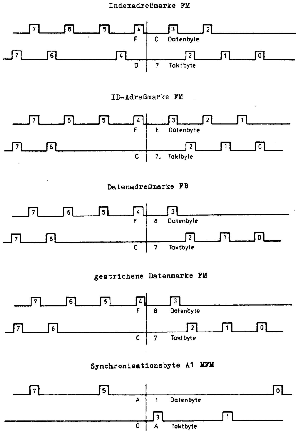
Abb. 4 Darstellung der Adreßmarken und des Synchronisationsbytes
