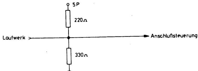
Abb. 2 Eingangsseitige Anpassung
