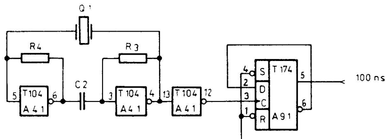
Abb. 6 Taktgenerator
