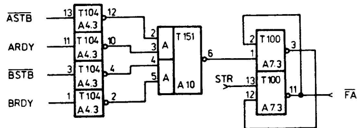
Abb. 11 Bildung des Signales Fehler
