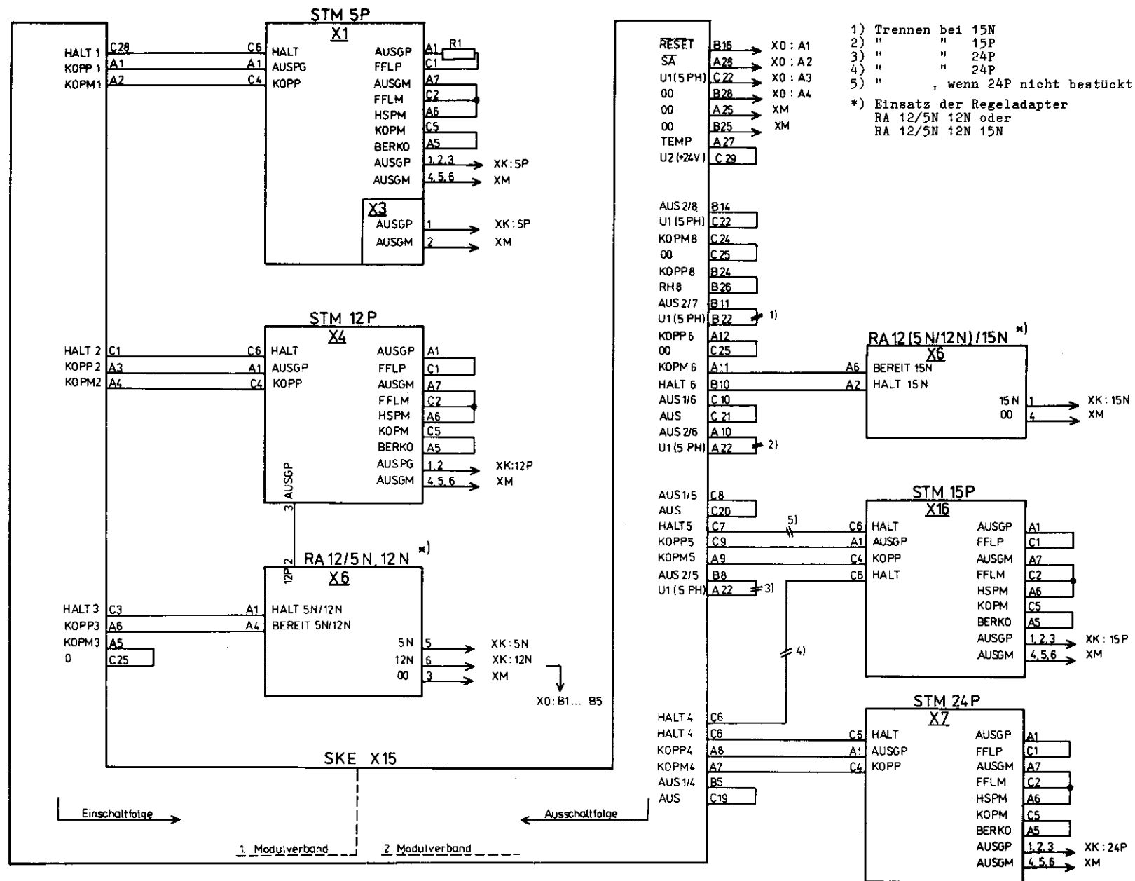
BSTM kpl. (Variante 028/029) Funktionsschaltplan (Steuersignale, Betriebsspannungen)
